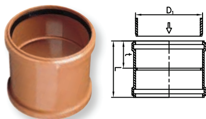
Spojka dvouhrdlá – KGMM
