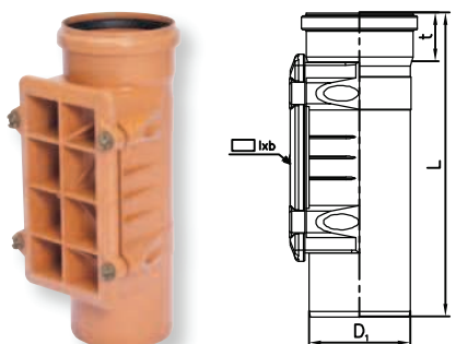
Čisticí kus šroubový – KGRE
