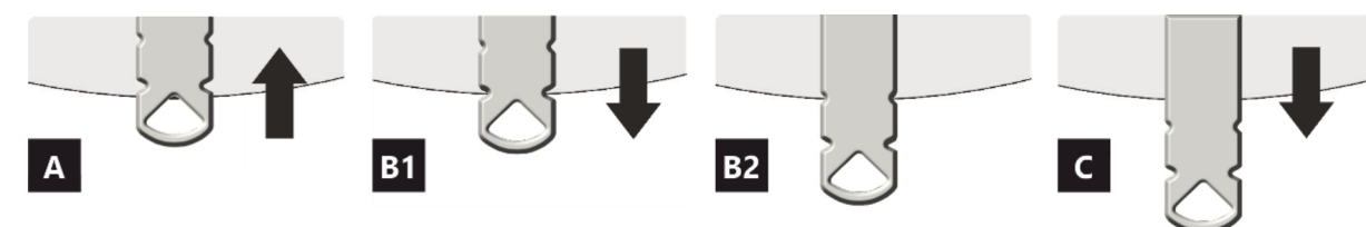
Рис. 9 Регулятор подачи воздуха – тип 5
