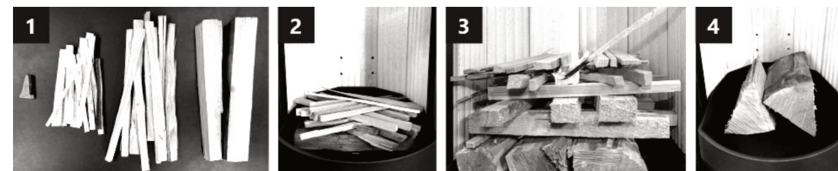
Rys. 4 Procedura przygotowania drewna w komorze spalania
