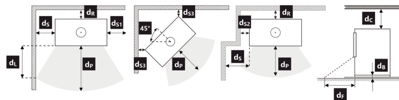
Obr. 2 Bezpečnostné odstupy od horľavých materiálov
