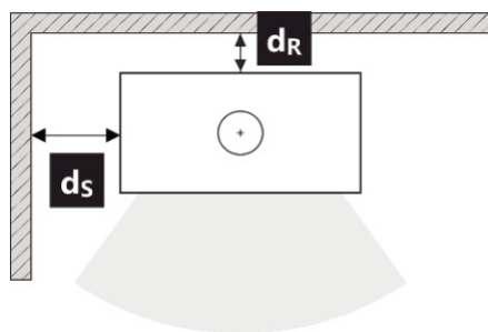
Obr. 3 Bezpečnostní odstupy od nehořlavých materiálů
