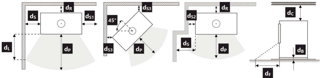
Rys. 2 Odległość od materiałów łatwopalnych
