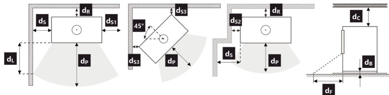
Obr. 2 Bezpečnostní odstupy od hořlavých materiálů
