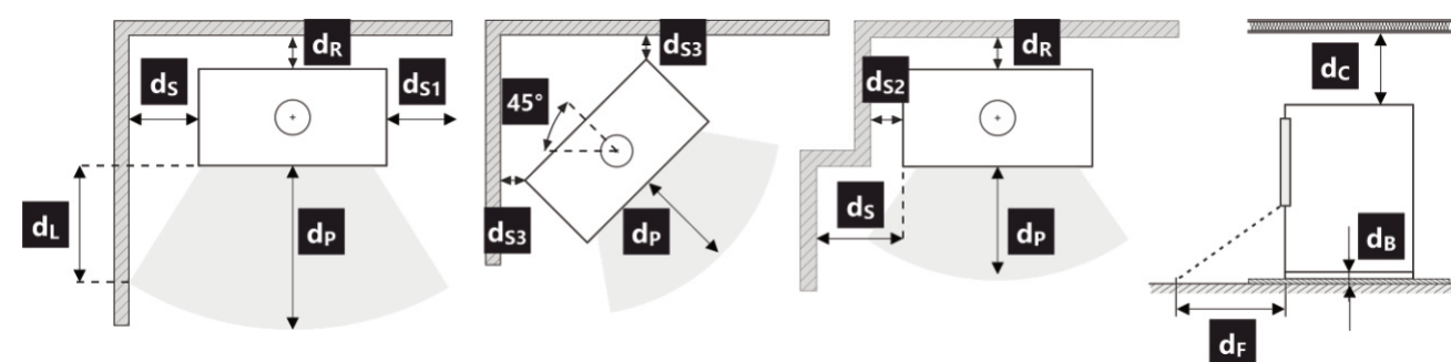
Kép 2 Távolság gyúlékony anyagoktól
