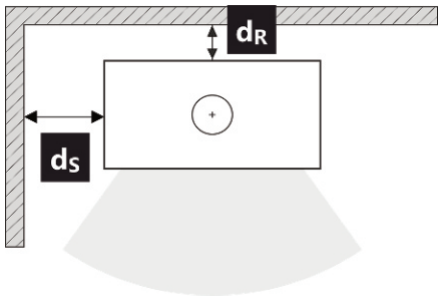
Рис. 3 Расстояние от невоспламеняющихся материалов
