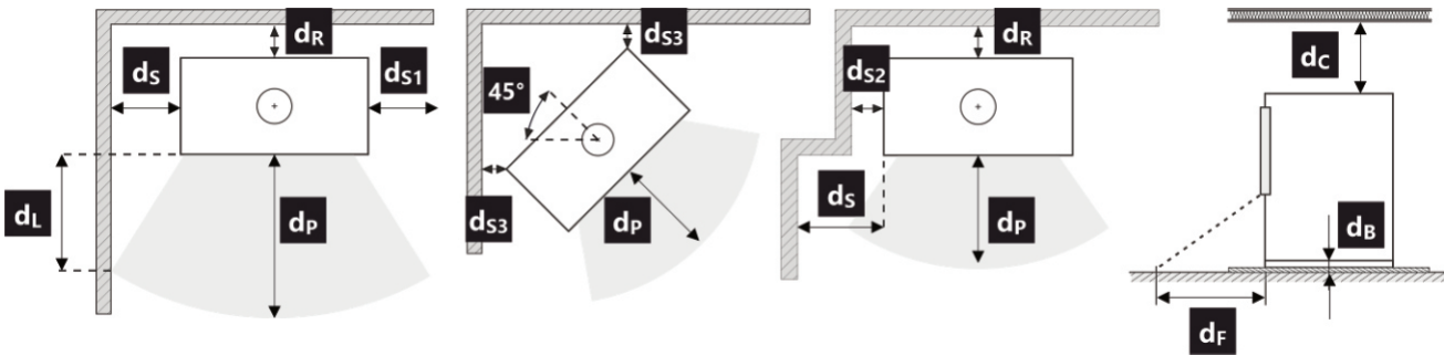
Рис. 2 Расстояние от горючих материалов
