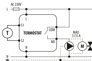
b) Schéma připojení k čerpadlu/pohonu ventilu
