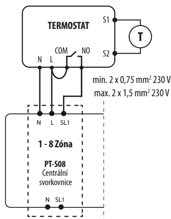
c) Schéma připojení k centrální svorkovnici
