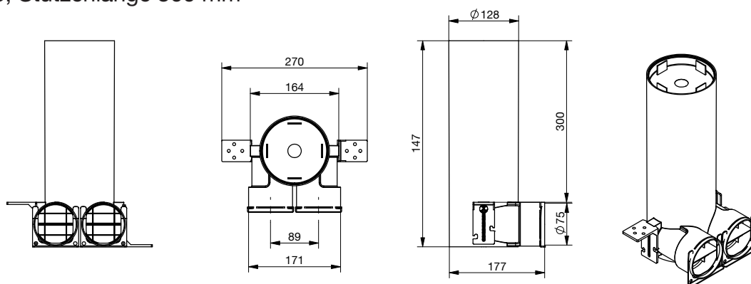
TVA-P 90, Stutzenlänge 300 mm
