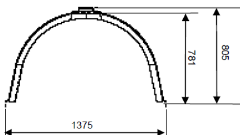
Rozměry jednotlivých prvků tunelu AS-KRECHT
