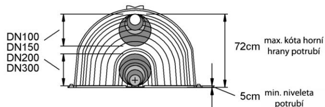
Rozměry jednotlivých prvků tunelu AS-KRECHT
