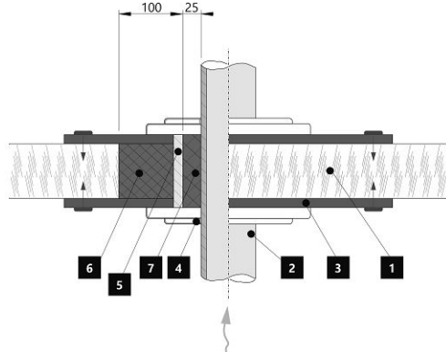
Прокладка дымовой трубы через стену из горючего материала
