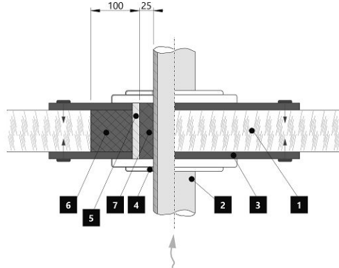
Прход дымовай трубы праз сцяну з гаручага матэрыяла
