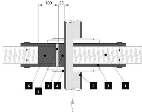
Прход дымовој трубы чeрeз стeну из горючeго матeриалa
