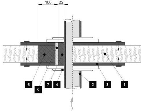
Прход дымовой трубы через стену из горючего материала
