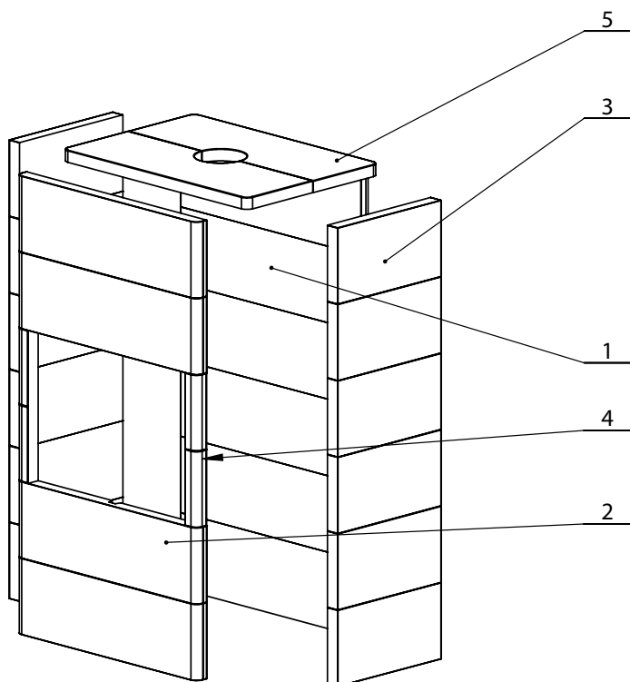
Schéma betonové obestavby
