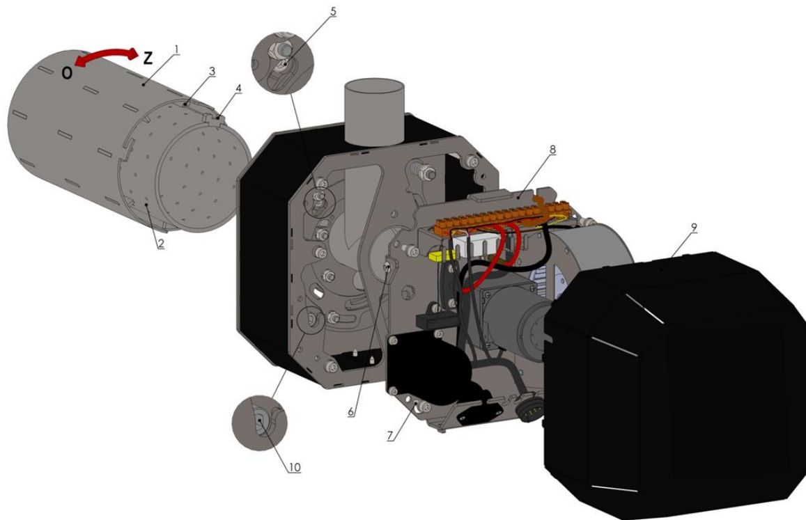
Obr. č. 22 Čištění trubkové provzdušňovací rotační komory – pohled 1
