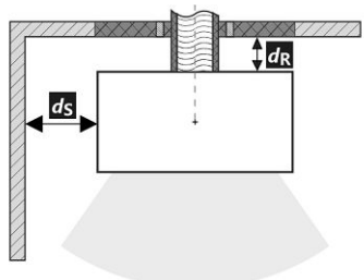
Заднее подключение дымохода (изолированное)
