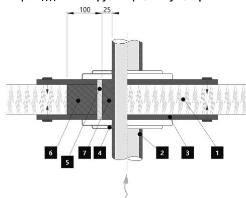
Прогон дымовой трубы через стену из горючего материала
