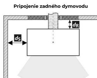
Prechod dymovodu cez stenu z horľavého materiálu
