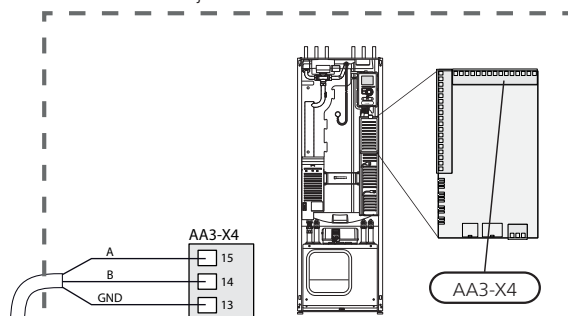
EB100 - nadřízená jednotka
