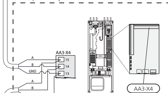
EB101 - podřízená jednotka 1
