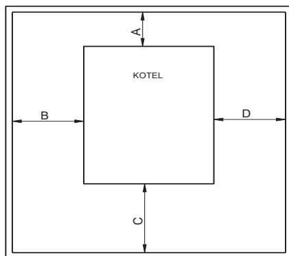
Obr. 5 Umístění kotle v kotelně.
