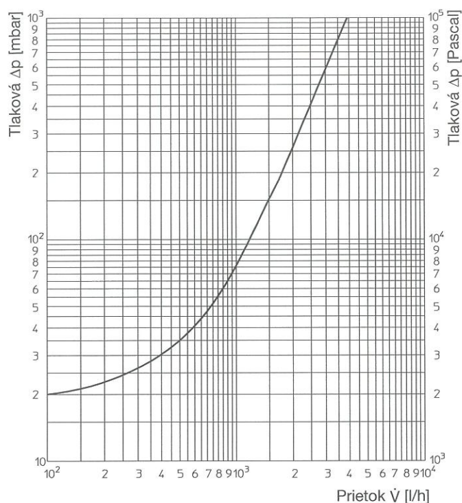
Prietokový diagram Regumat RTA
