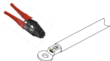
Krimpovací kleště
