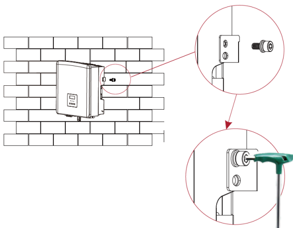
Vnitřní šestihranný klíč (utahovací moment 1,2 +/-0,1 Nm)
