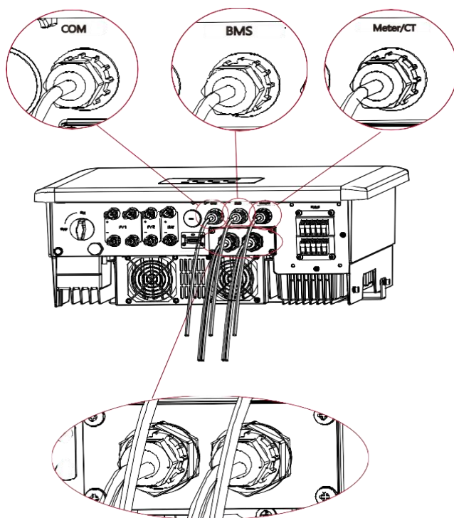
Vodotěsný konektor s RJ 45
