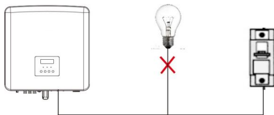
Nesprávné připojení zátěže k měniči
