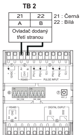
Rozhraní měřidla
