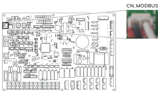
Vnitřní DPS
