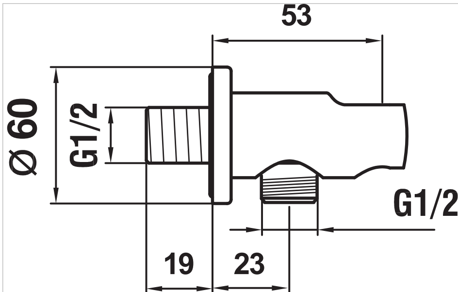
Technické výkresy
