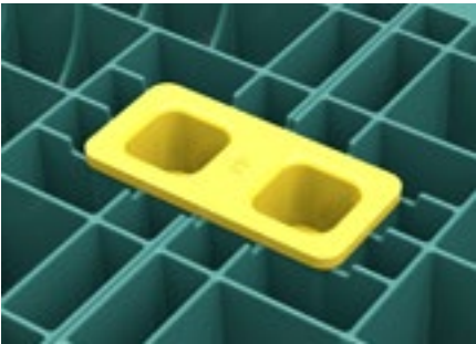
Spojka bloku jednovrstvá pro montáž do stropní desky u půlvrstevých a horního základního prvku u jednovrstvých galerií
