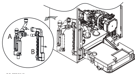
Obr.59 Demontáž sifonu
