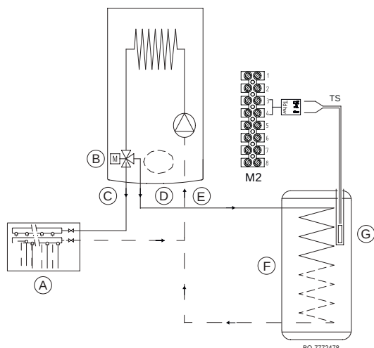
Obr.88 Pripojenie zásobníka TUV
