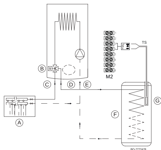
Obr.26 Připojení zásobníku TV
