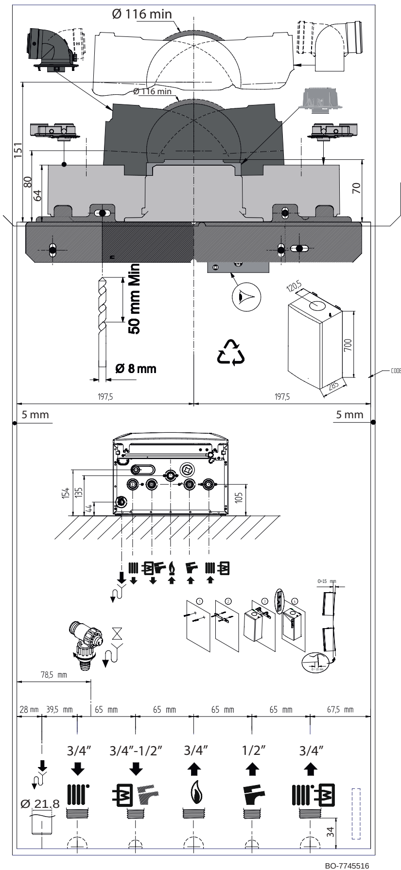
Obr.75 Papierová šablóna kombinovaného modelu Vykurovanie + Teplá úžitková voda
