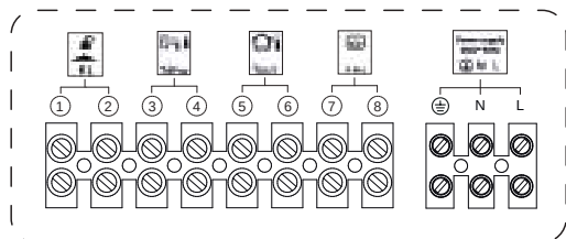
Obr.38 Připojení desky kotle
