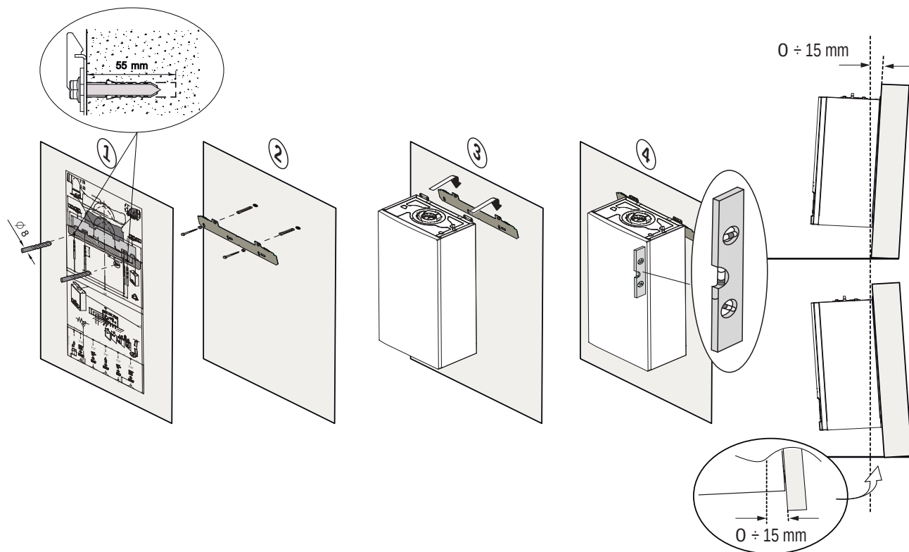
Obr.85 Inštalácia na stenu
