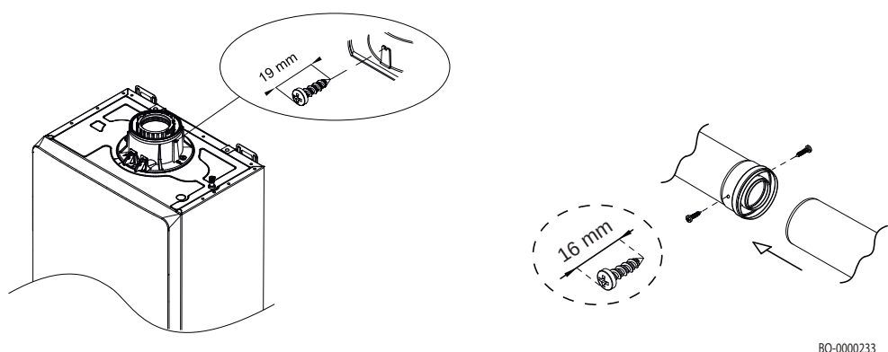
Obr.30 Upevnění věže koaxiálního odvodu spalin
