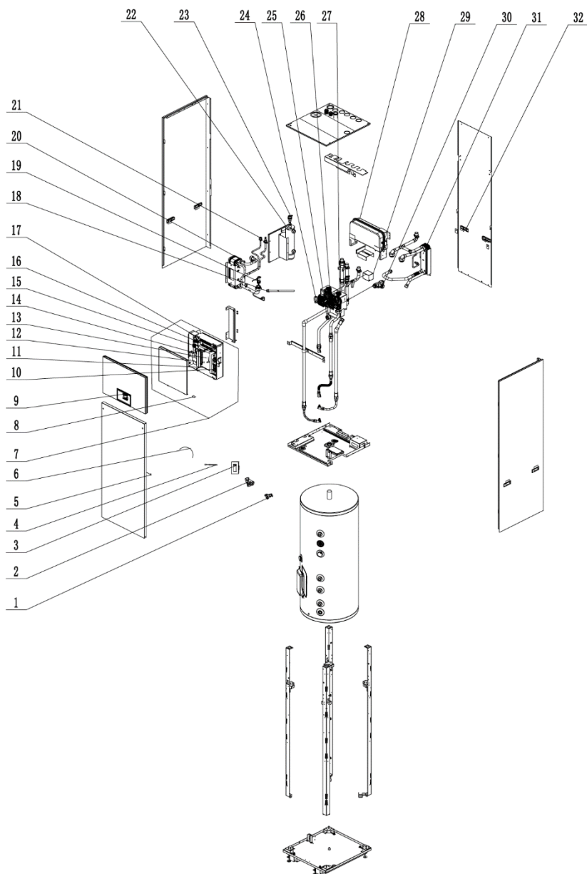
Seznam dílů GRS-CQ8.0PdG/NhH2-M(I), GRS-CQ10PdG/NhH2-M(I)
