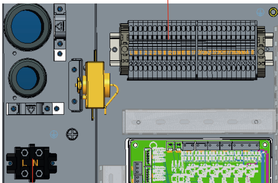
Svorkovnice XT1
