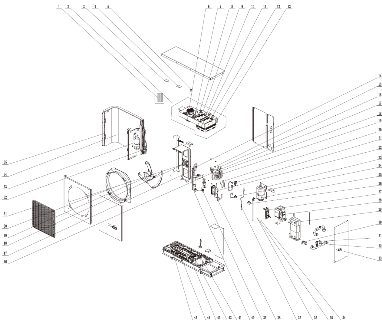
Seznam dílů GRS-CQ4.0Pd/NhG-K, GRS-CQ6.0Pd/NhG-K, GRS-CQ8.0Pd/NhG-K
