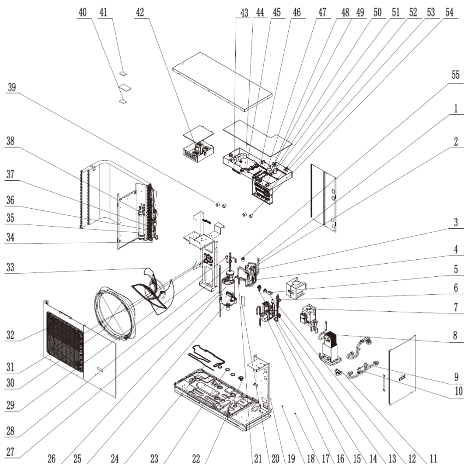
Seznam dílů GRS-CQ10Pd/NhG-M, GRS-CQ12Pd/NhG-M, GRS-CQ14Pd/NhG-M, GRS-CQ16Pd/NhG-M
