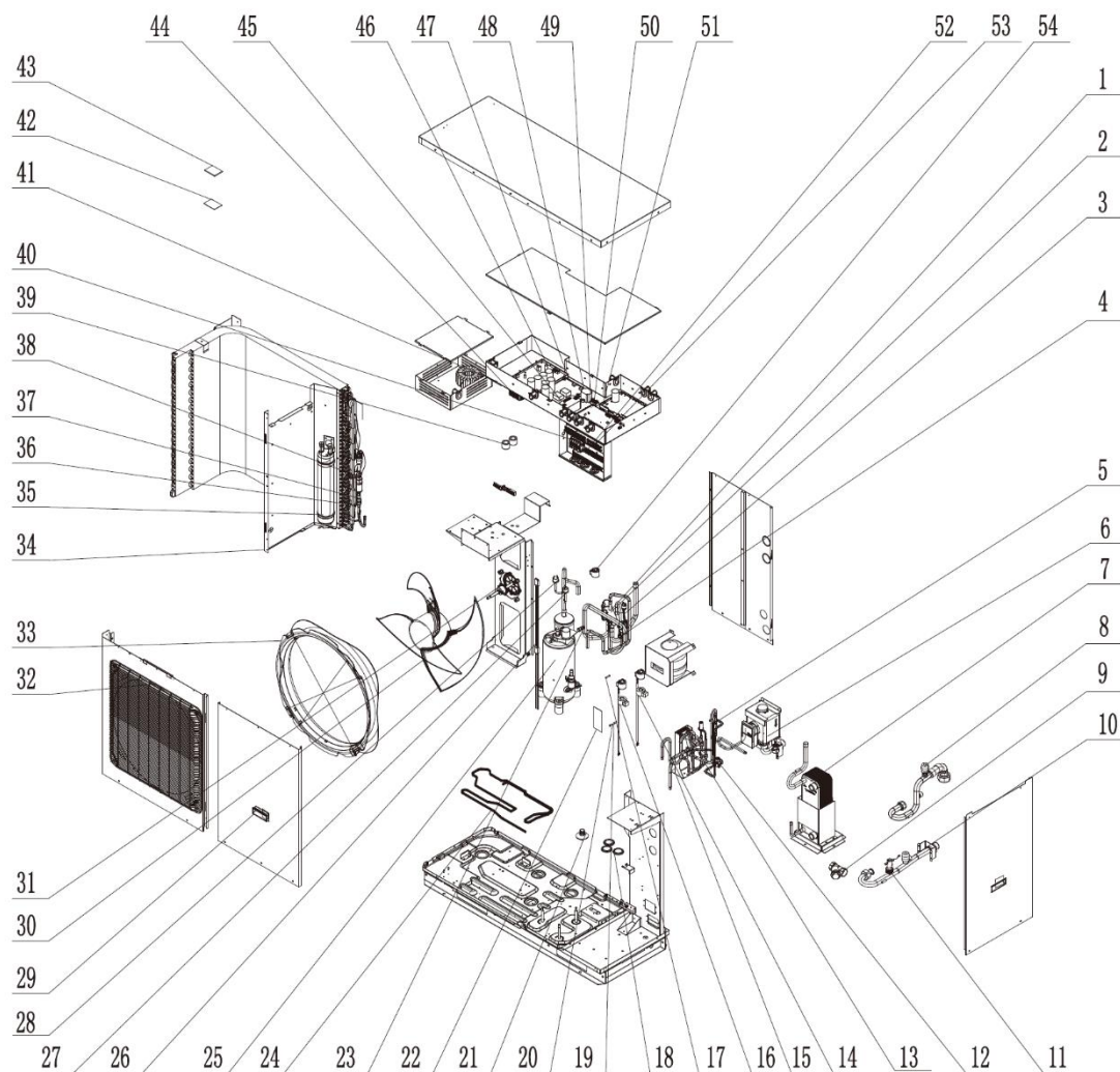
Seznam dílů GRS-CQ10Pd/NhG-E, GRS-CQ12Pd/NhG-E, GRS-CQ14Pd/NhG-E, GRS-CQ16Pd/NhG-E
